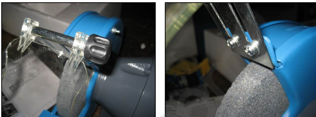
Figura 5 – Montaggio degli schermi di protezione.
