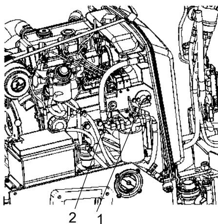
Fig. Vano batteria 1. Interruttore di isolamento batteria 2. Presa di alimentazione, 12 V
