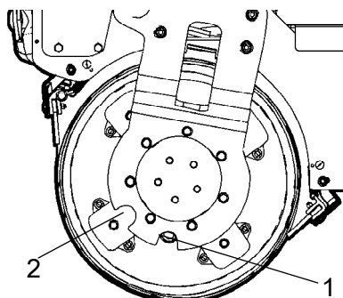
Fig. Tamburo, lato vibrazione
