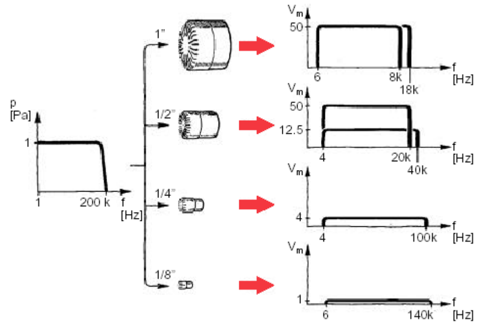
Sensibilità e risposta in frequenza in funzione delle dimensioni della capsula
