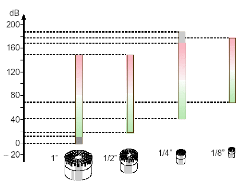
Range dinamico e dimensioni della capsula
