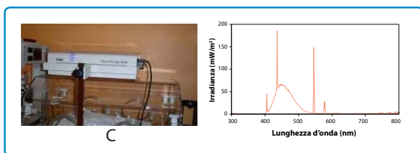
Immagini di dispositivi fototerapeutici insieme agli spettri di uscita misurati. (A) Waldmann UV 7001 UVB. (B) Waldmann UV 181 BL. (C) Dräger PhotoTherapy 4000
