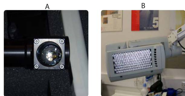
Immagini di sorgenti per terapia fotodinamica. (A) UV-X. (B) Aktilite CL128
