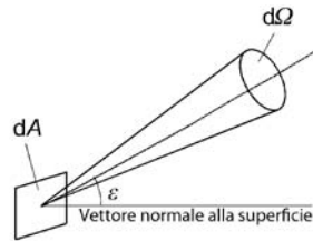
Schema della definizione di radianza.
